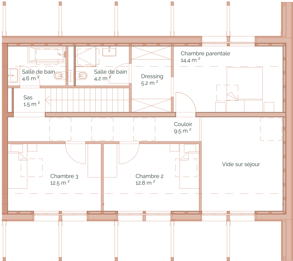
1er étage
